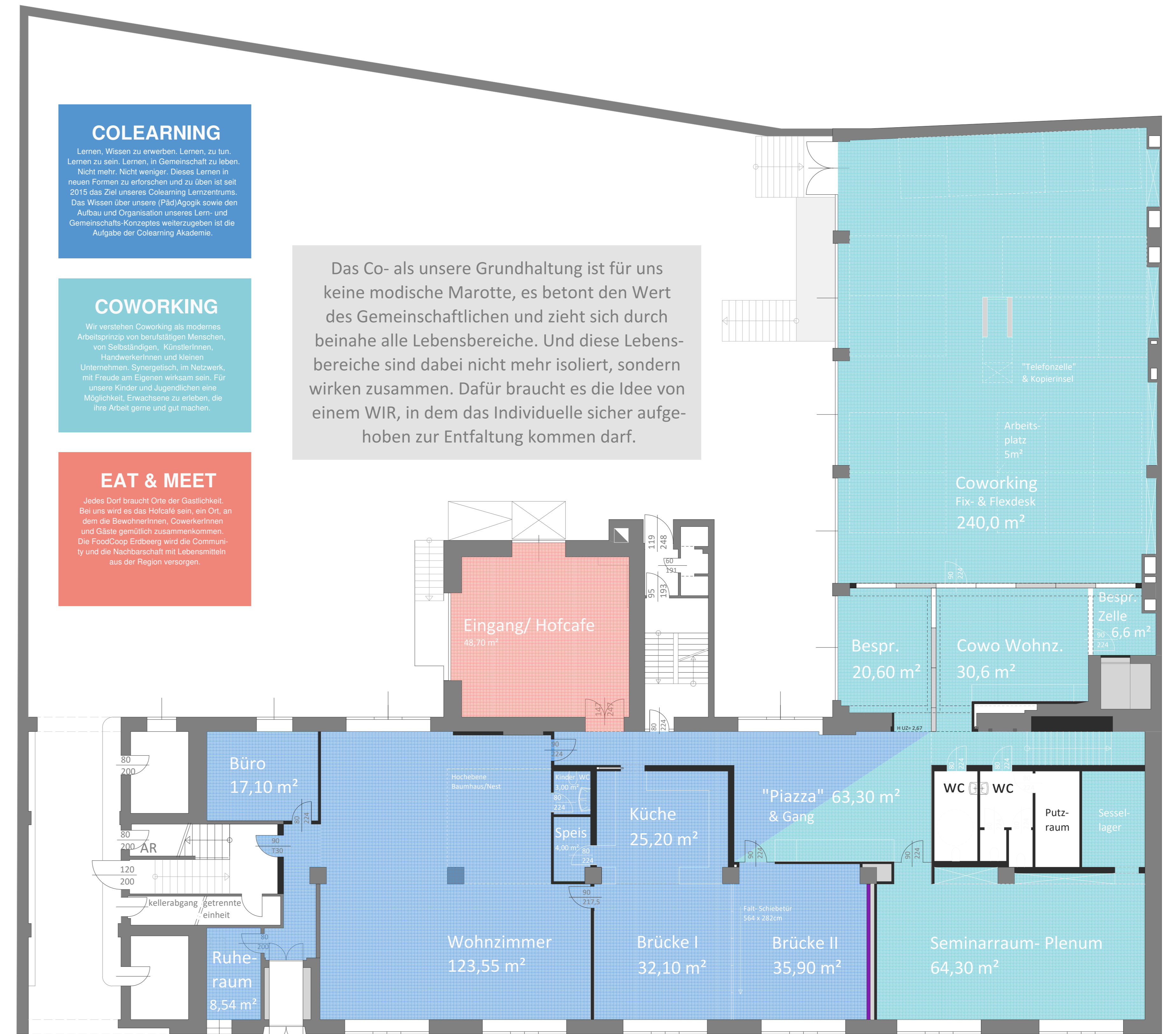
ERDGESCHOSS 1:100
